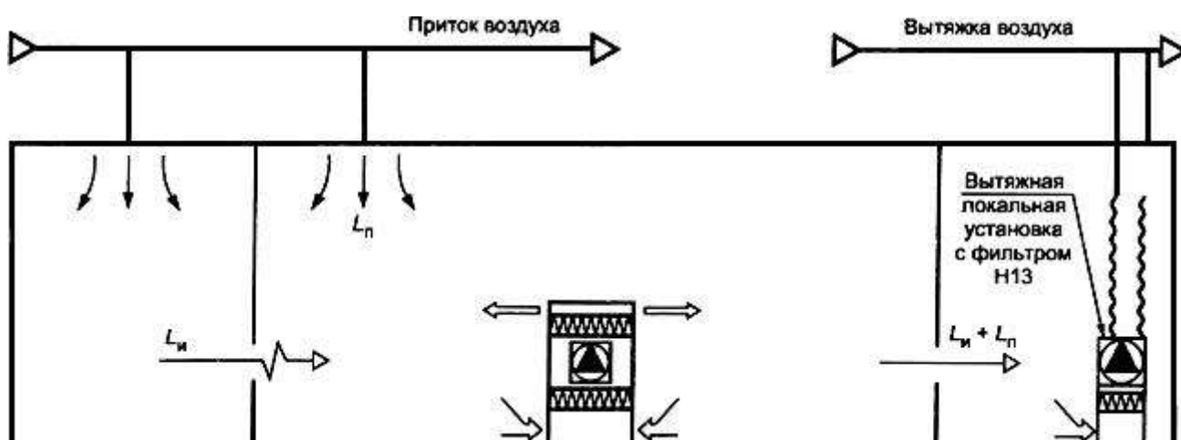
Рисунок 3 - Применение автономного устройства очистки воздуха в помещениях группы 5 (изоляторах)
